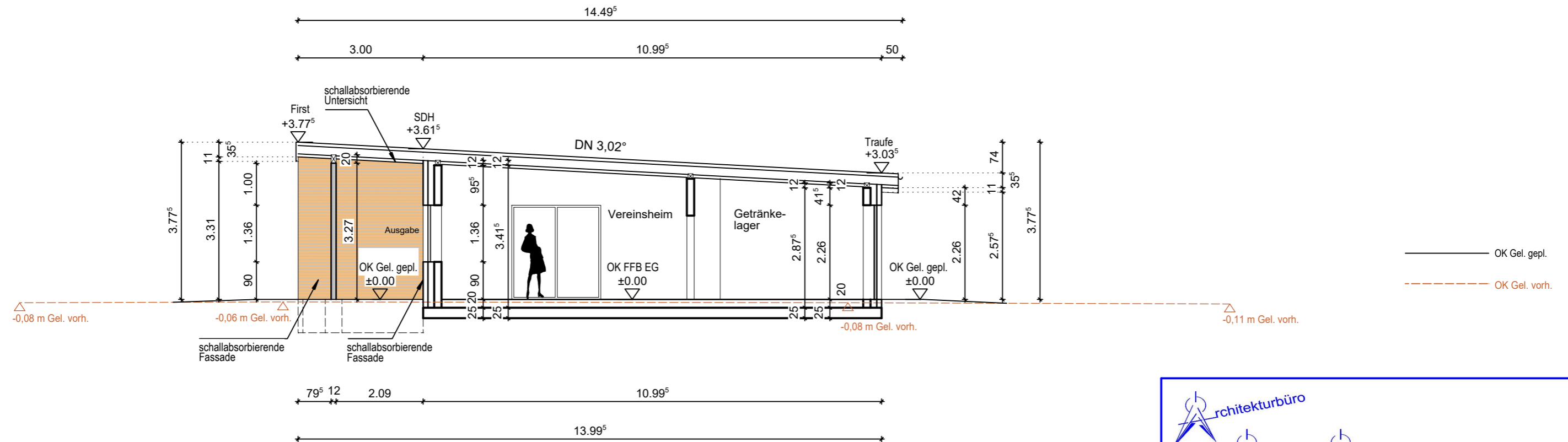
Schnitt A-A
